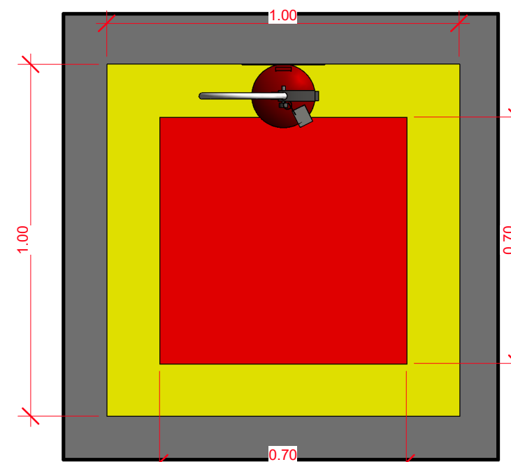
5 Extintores 3
