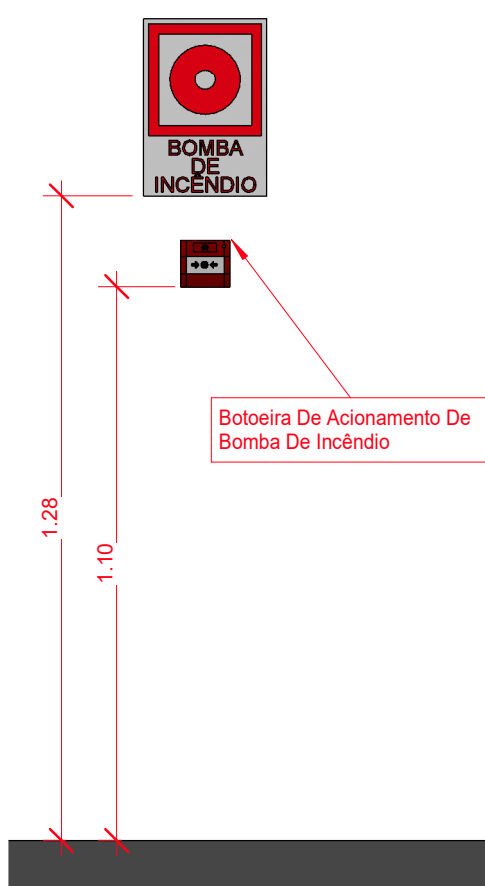
7 Detalhe 02 1 : 15
