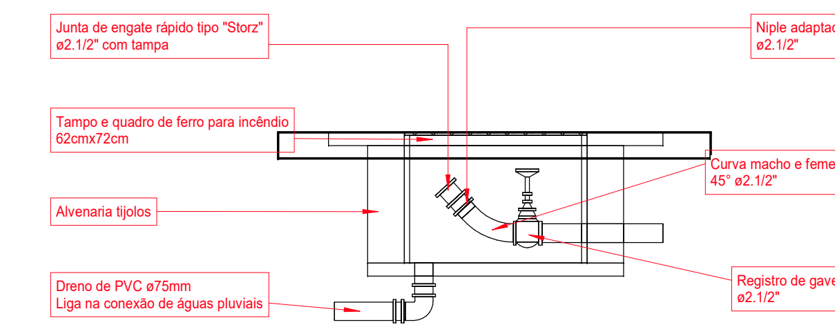
17 Hidrantes de recalque 2
