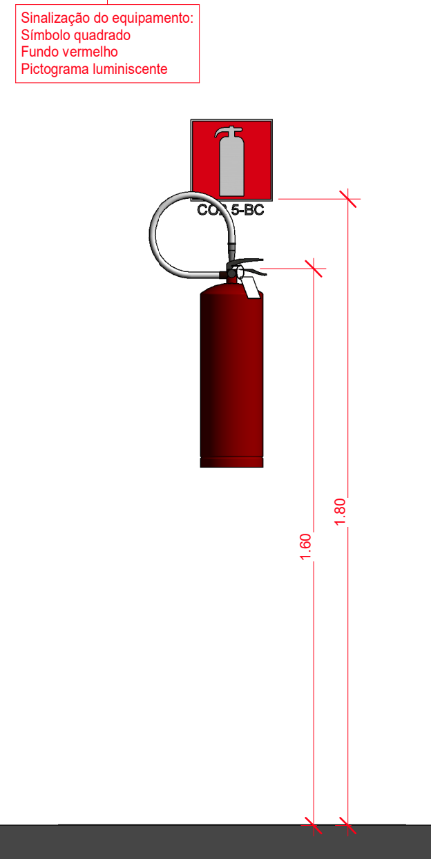
8 Extintores 2 1 : 15
