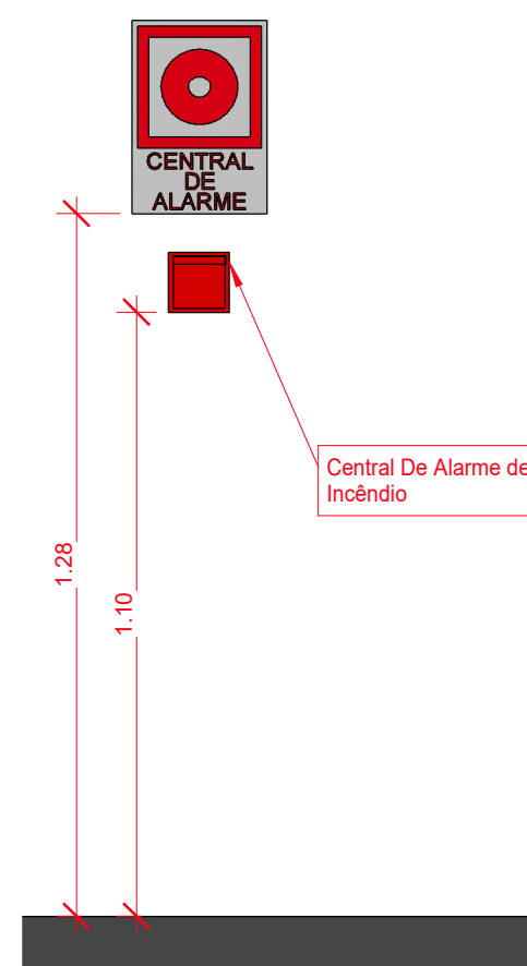
2 Detalhe 03 1 : 15
