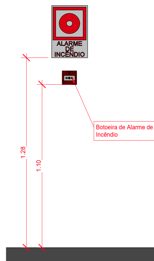
15 Detalhe 01 1 : 15
