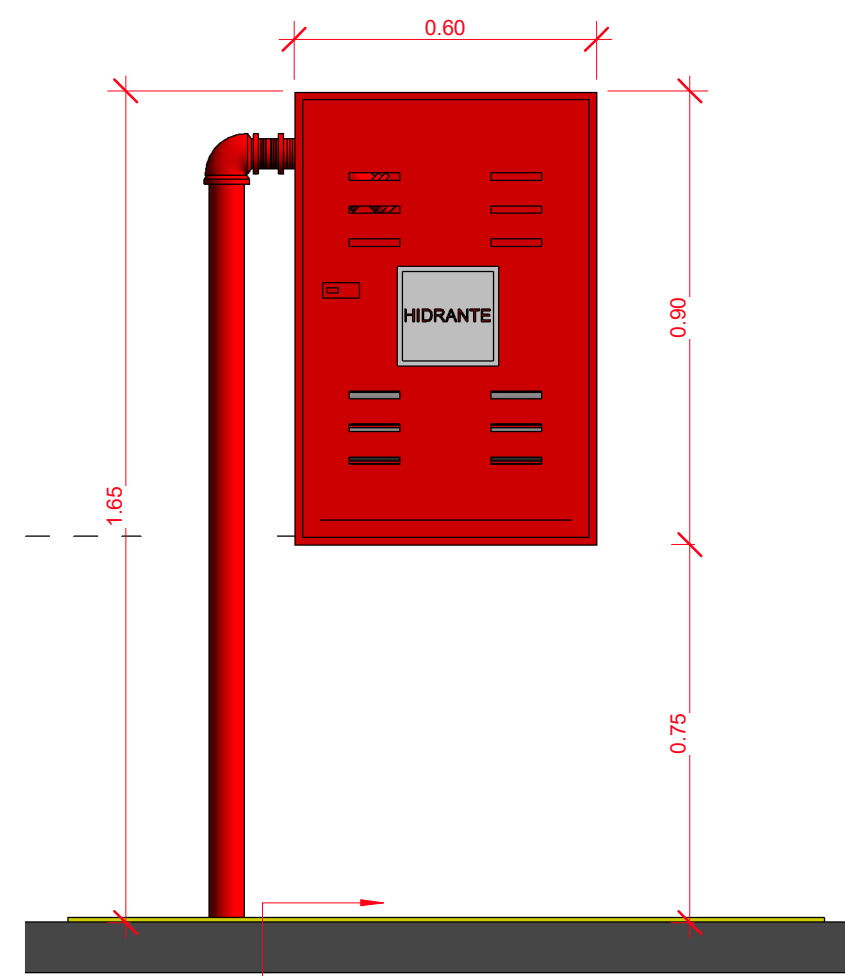
11 Hidrantes 2 1 : 15
