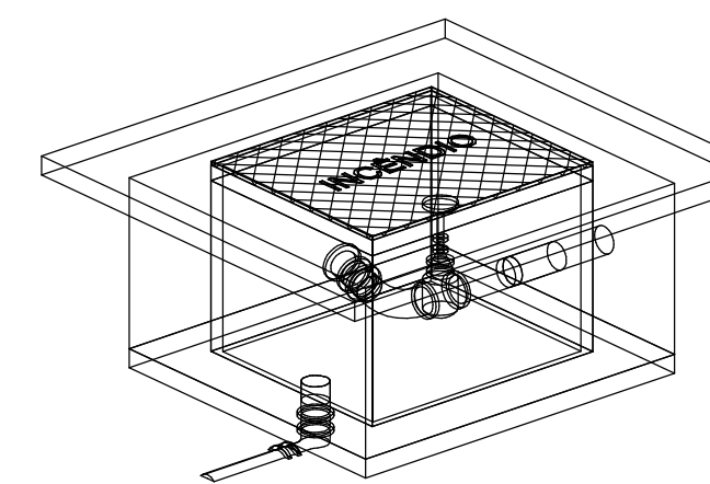
6 Hidrantes de recalque 1
